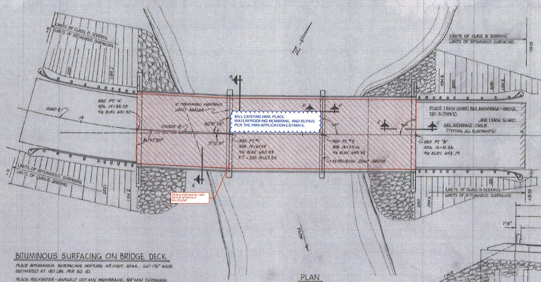
PLAN SCALE: 1\"/>
