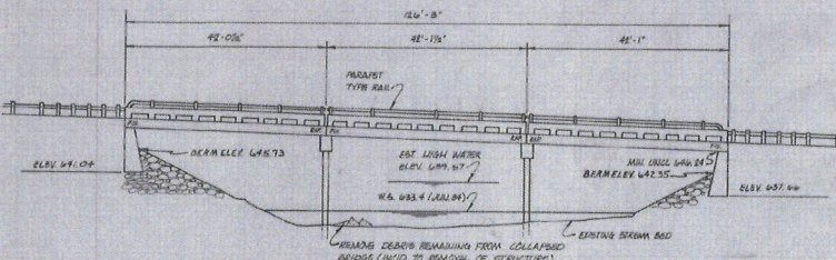
ELEVATION SCALE: 1\"/>
